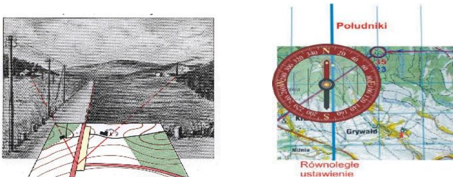
Rys. 125. Orientowanie mapy
