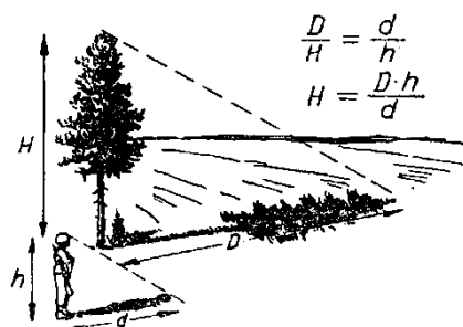
Rys. 121. Pomiar wysokości
